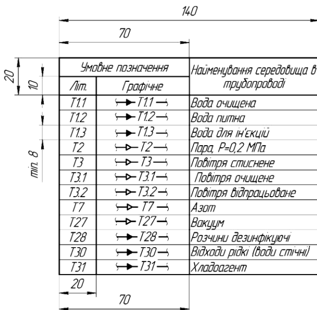
Рис. 3.1. Приклад оформлення таблиці умовних позначень трубопроводів
