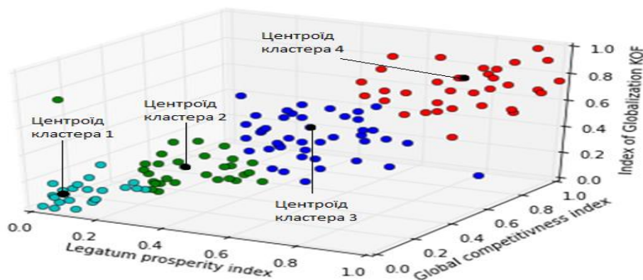
Рис. 2.4. Кластеризація країн за станом їх економічного розвитку, 2013–2023 рр. Джерело: розроблено автором на основі [5, 6 ,9, 12].
