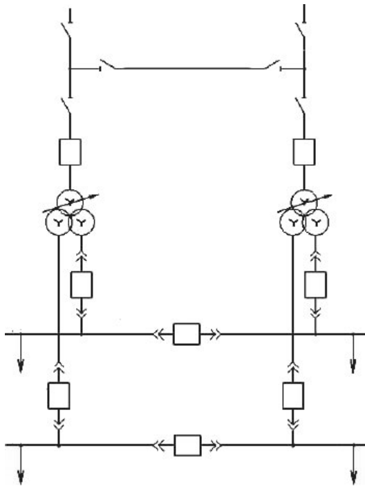
Рисунок 3 - Спрощена електрична схема підстанції
