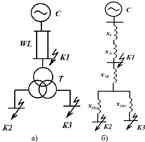
Рисунок 4 - Розрахункова схема (а) та схема заміщення (б)
