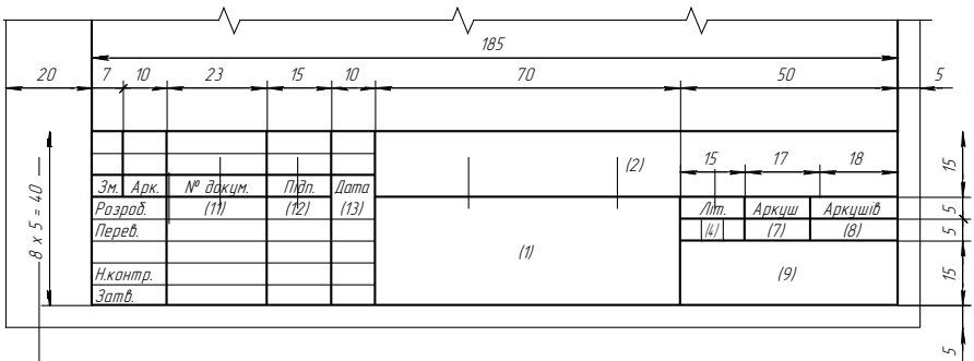
Рисунок 2 – Основний напис першого аркуша текстового документа
