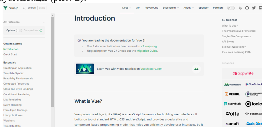
Рис. 2. Документація Vue.js [2]
