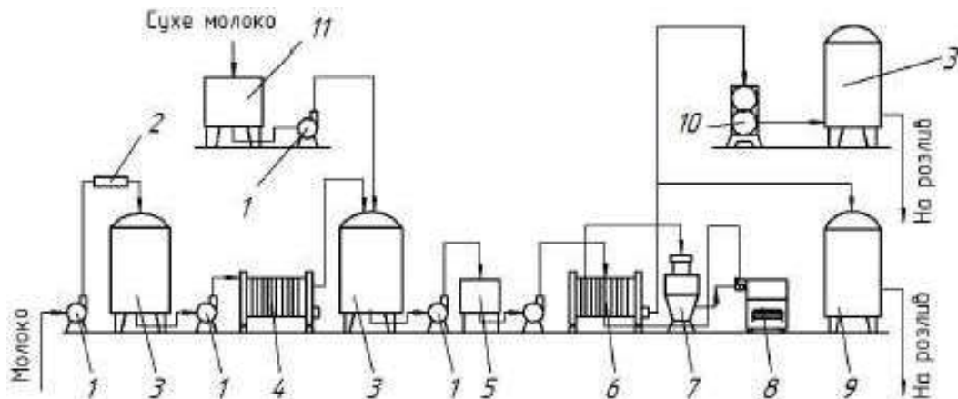
Рис.1 Машино-апаратурна схема виробництва пастеризованого молока
